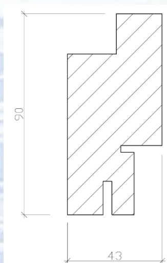
Сечение лутки в моделях ALL-GLASS
