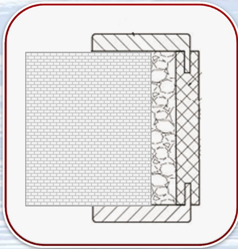
Рис.1 Фальшкоробка
