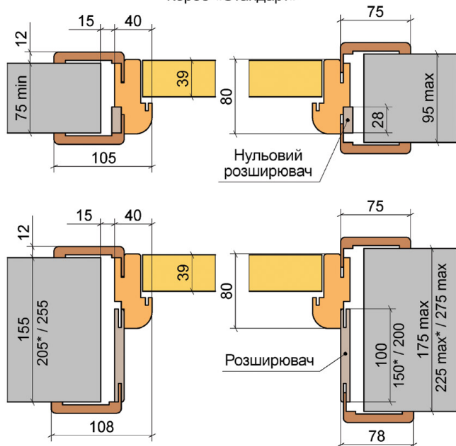
Короб «Стандарт»
