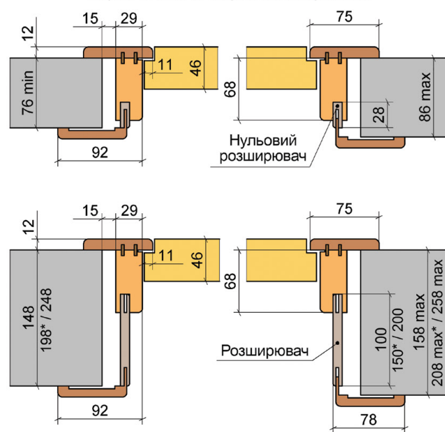
Короб «INSIDE» зворотного відкривання
