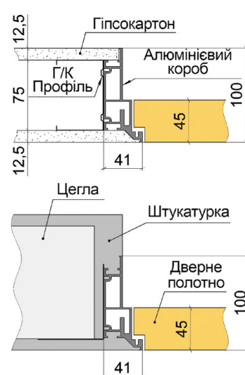
Алюмінієвий короб «преміум» зворотного відкривання
