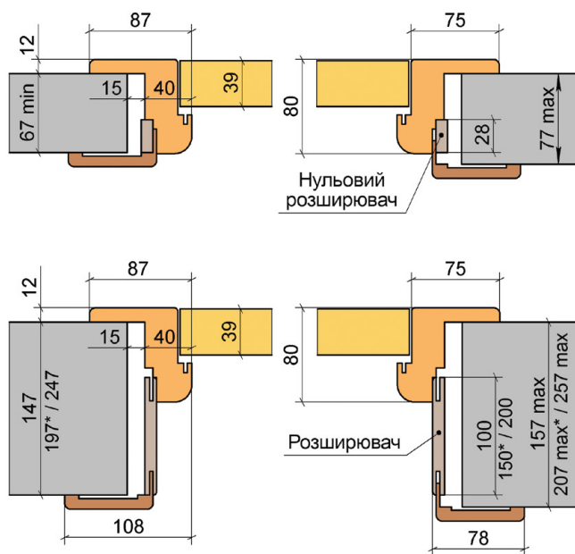
Короб «Еліт»
