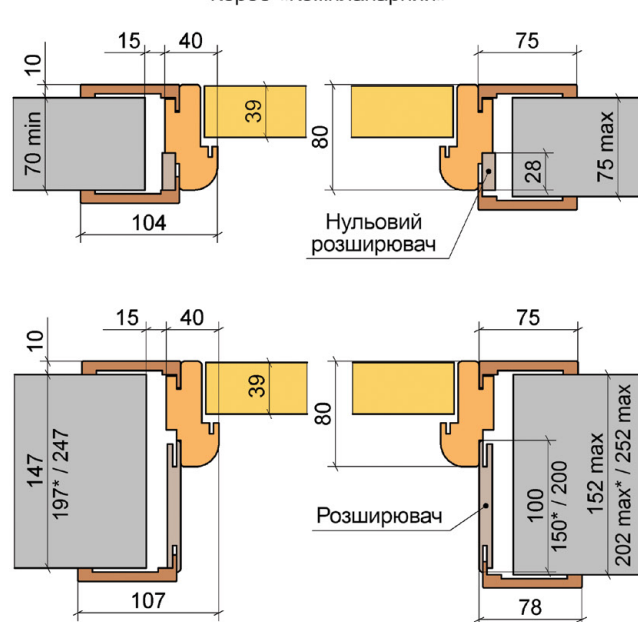
Короб «Компланарний»
